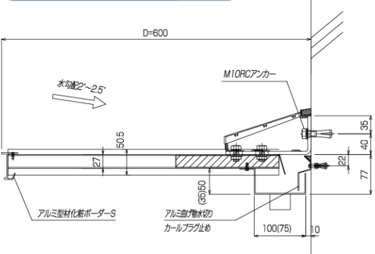
ALF2750-3-1S 断面図
