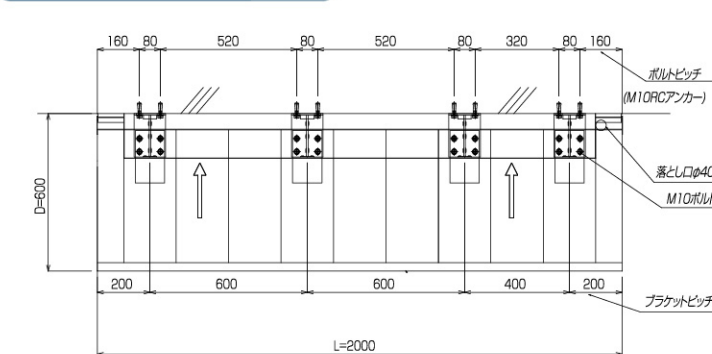
ALF2750-3-1S 平面図
