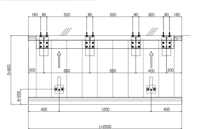
ALF2750-3-2R 平面図
