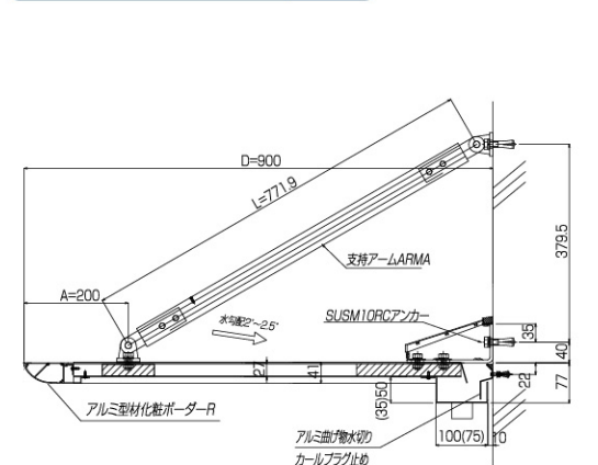
ALF2750-3-2R 断面図
