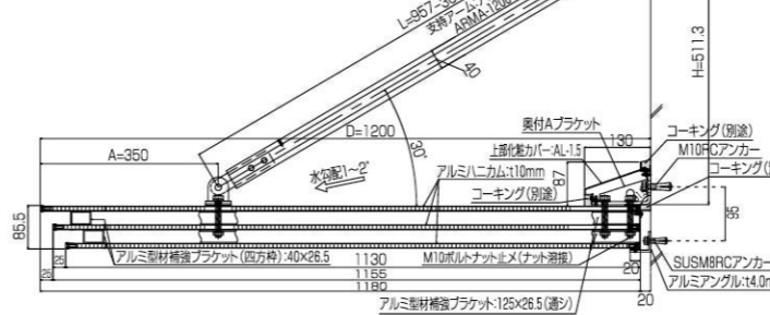
AFHV862-1200 断面図
