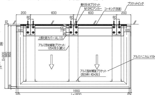
AFHV862-1200 L=1550 平面図
