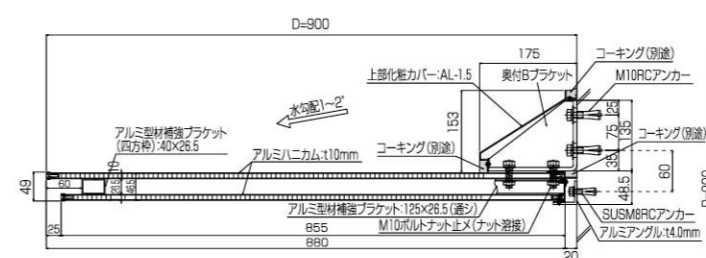
AFHV501-900 断面図
