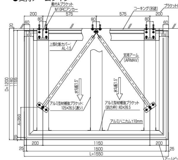
AFHV862-1200 L=1550 平面図
